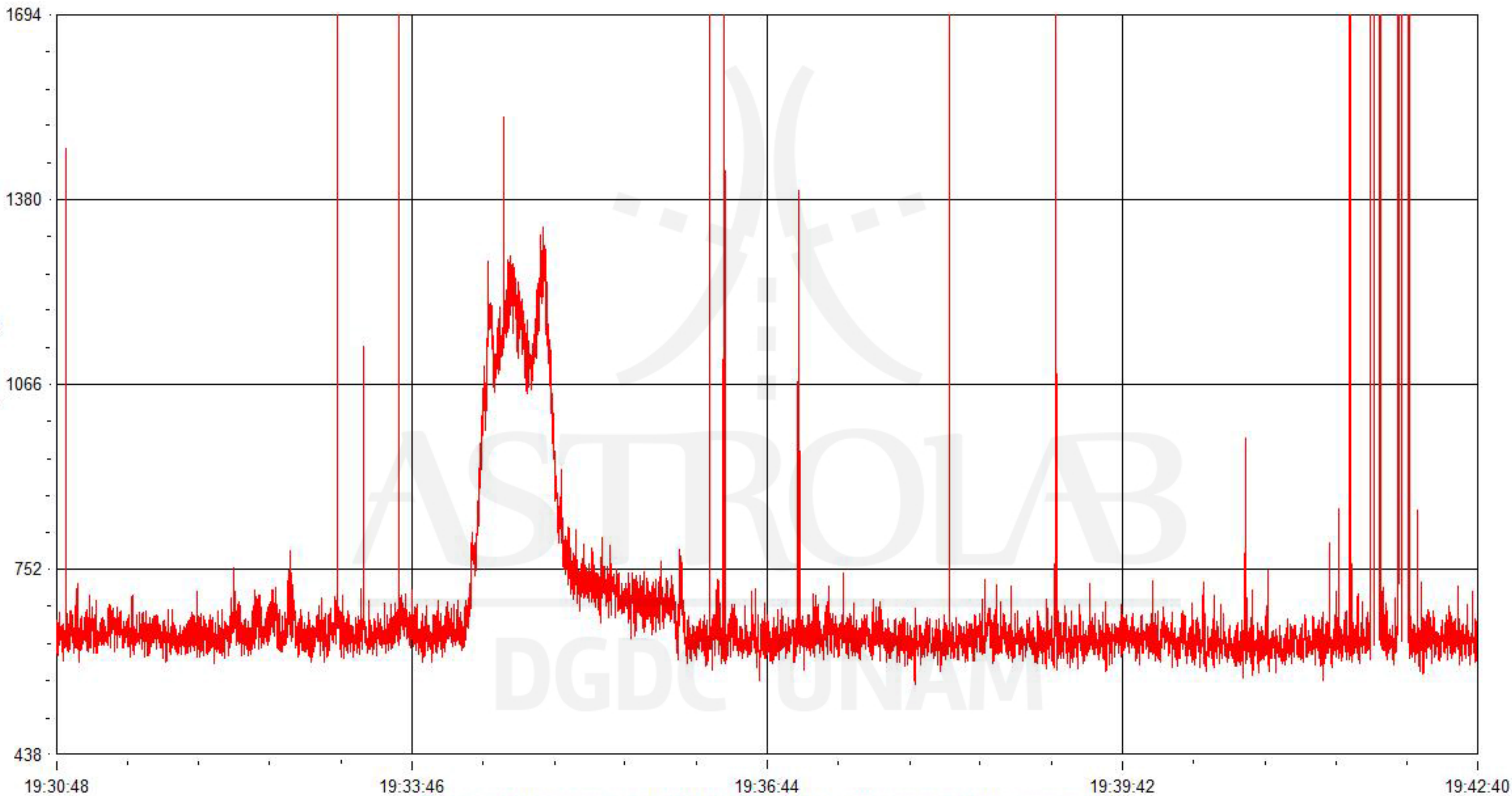
Radiotelescopio Astrolab (Tiempo Universal )
